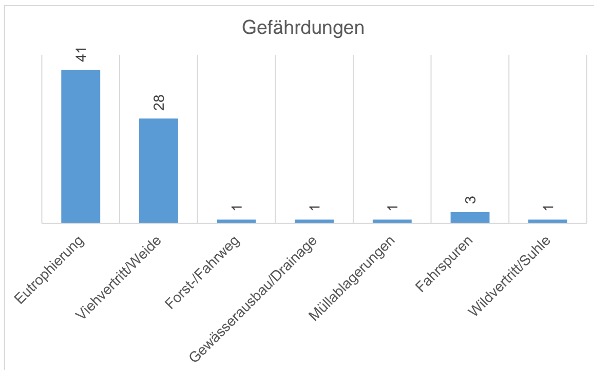
Abb.: Festgestellte Gefährdungen bei den Quellen im Untersuchungsgebiet
